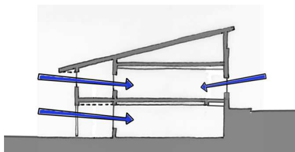
Principes d'éclairage des salles de l'école élémentaire
